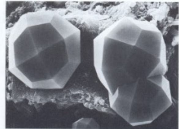
Figura 2.1 Immagine al microscopio elettronico a scansione (SEM) di tre cristalli perfettamente formati del minerale analcima, \text{NaAlSi}_3\text{O}_8 \cdot \text{H}_2\text{O} (Ischia, Italia). Questi cristalli mostrano un'unica forma, il trapezoedro, che riflette l'elevata simmetria del sistema cubico. Il trapezoedro è formato da 24 facce a forma di trapezio (da Gottardi, G. e Galli, E., 1985, Natural Zeolites , Springer-Verlag, New York, riproduzione autorizzata).
