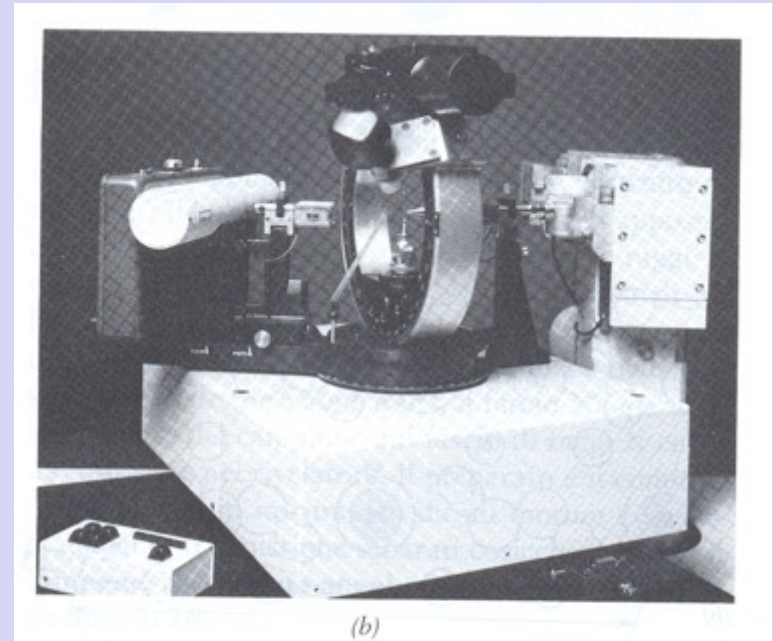
Figura 7.41 (a) Schema del diffrattometro a cristallo singolo modello P4 prodotto dalla Siemens Industrial Automation, Inc. (b) Vista ravvicinata di un goniometro a quattro cerchi per il controllo dell'orientamento di un cristallo singolo (al centro dell'immagine). Sul lato destro è posizionato il tubo a raggi X e sul lato sinistro il contatore di raggi X, del tipo a scintillazione (per concessione di Siemens Industrial Automation, Inc., Madison Wisconsin).
