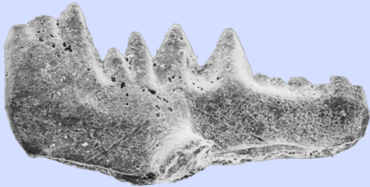
conodonti
