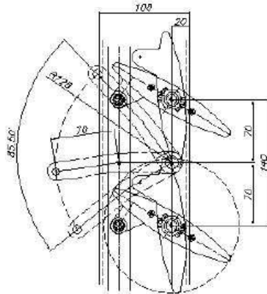
DETT. MANIGLIA interna SCALA 1:2
