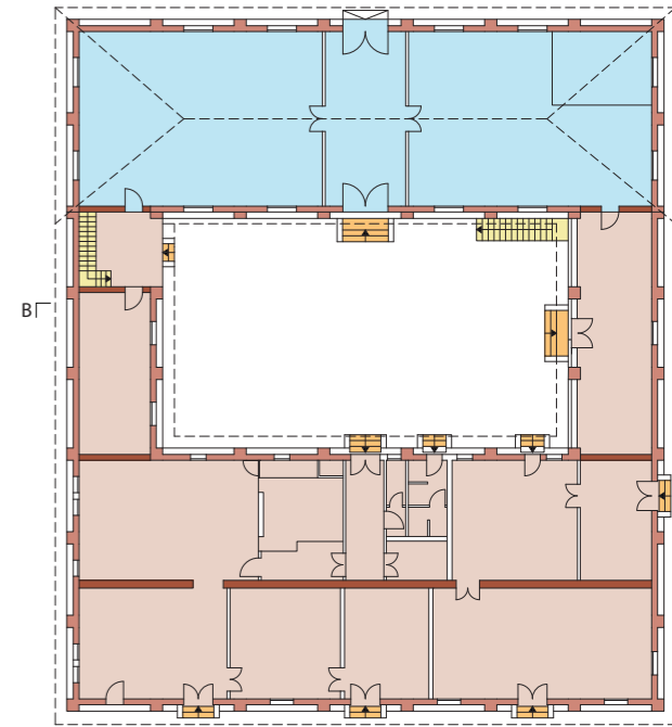
PIANTA DELLE STRUTTURE IN ELEVAZIONE DEL PIANO TERRA
