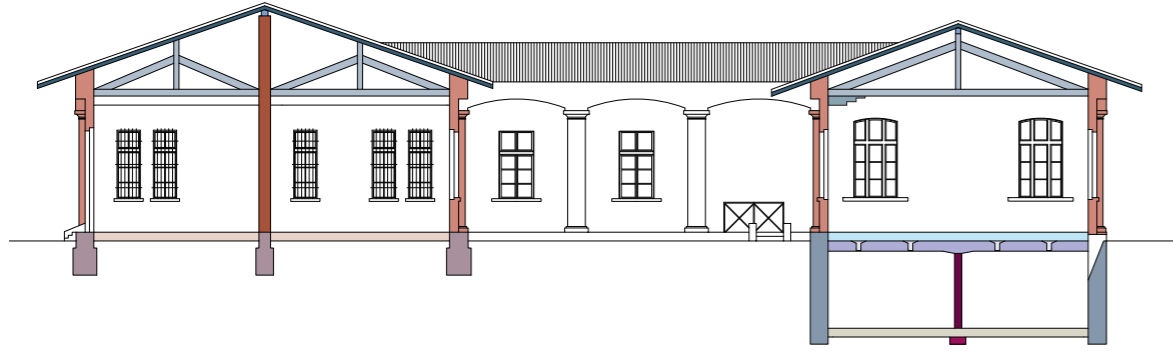
SEZIONE A-A'
