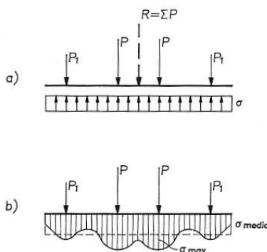
Differente andamento delle tensioni nel terreno lungo la trave in relazione al modello di calcolo adottato. a) Trave continua infinitamente rigida; b) Trave su suolo elastico.
