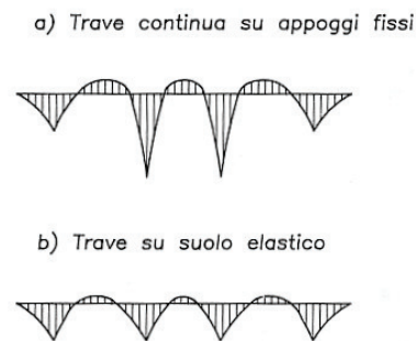
Differente andamento del diagramma dei momenti lungo la trave in relazione al modello di calcolo adottato. a) Trave continua su appoggi fissi; b) Trave su suolo elastico.
