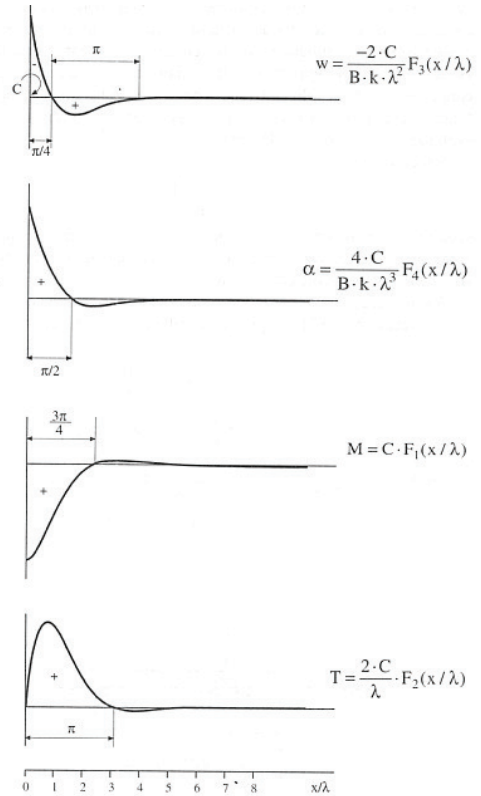
Fig. 9.6. Soluzioni per la trave di lunghezza infinita su suolo alla Winkler, caricata in una estremità da una coppia concentrata
