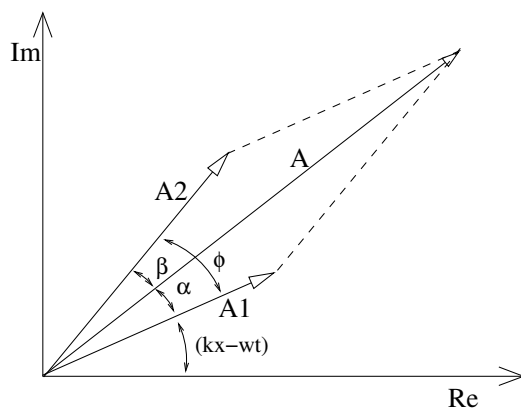
Figura 2: Interferenza tra due onde con differenza di fase costante
