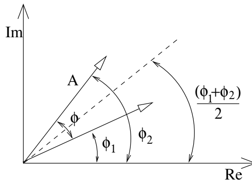
Figura 4: Battimenti
