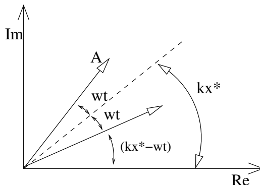
Figura 3: Onde stazionarie
