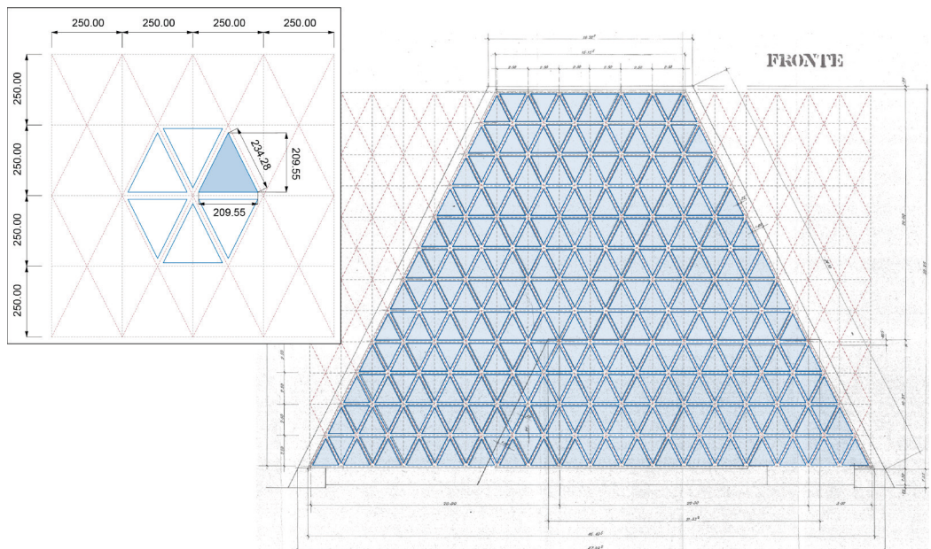
Fig. 7. Schema generativo sotteso all'orditura della maglia strutturale applicato al fronte dell'edificio. In dettaglio la definizione del modulo triangolare e le sue quote (elaborazione degli autori).
