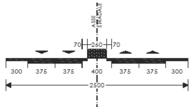
Soluzione base a 2+2 corsie di marcia
