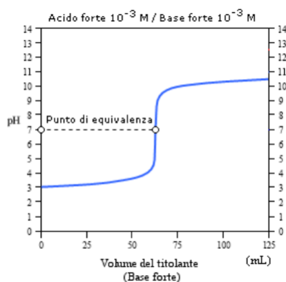
Curva di titolazione di un acido forte con una base forte
