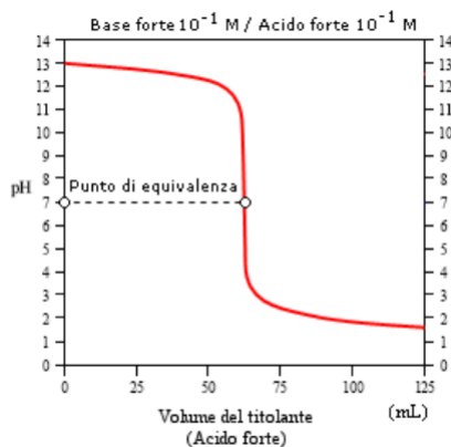
Curva di titolazione di una base forte con un acido forte
